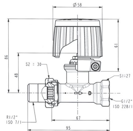
FJVR 15 (1/2") w wersji prostej
