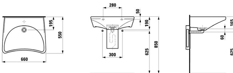
Rysunek techniczny
