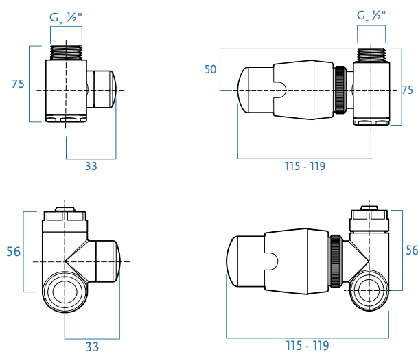
Układ zaworu typ PRAWY podłączenie [11]
