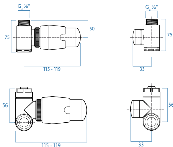
Układ zaworu typ LEWY podłączenie [11]
