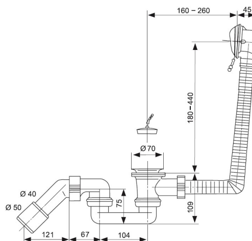
Rysunek techniczny
