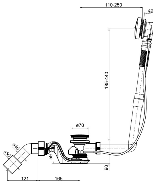
Rysunek techniczny
