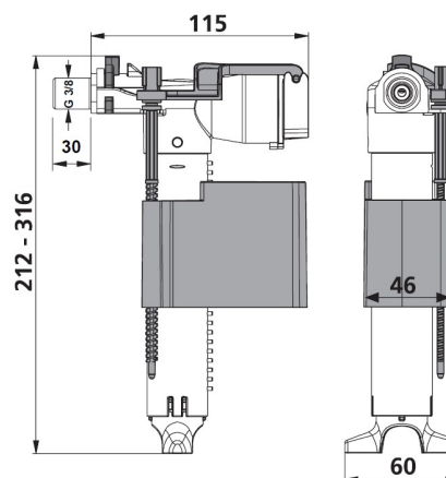
Rysunek techniczny
