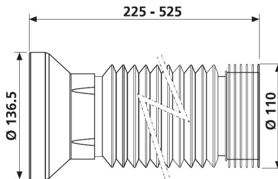
Rysunek techniczny
