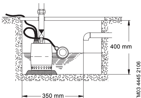
Rys. 2 Min. wymiary studzienki dla Unilift KP-A
