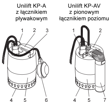
Rys. 1 Pompa z łącnikiem poziomym
