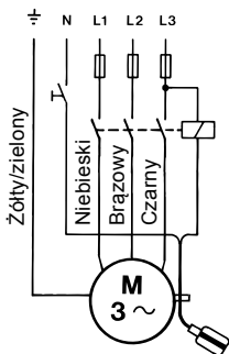
Rys. 8 Schemat elektryczny
